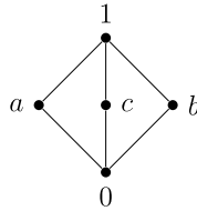
Fig. 1. Lattice M_3 .
